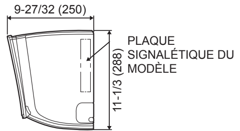
VUE LATÉRALE
