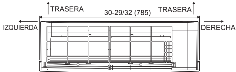
VISTA SUPERIOR
